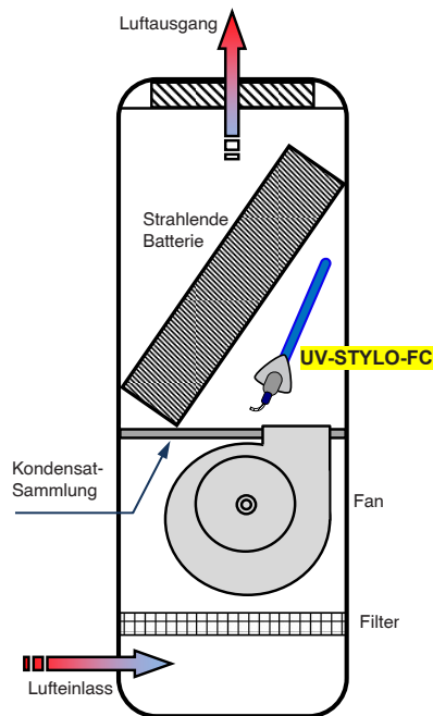
Anwendungsdigramm
